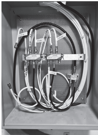
Hausanschlusskasten Koaxial-Kabelnetz
