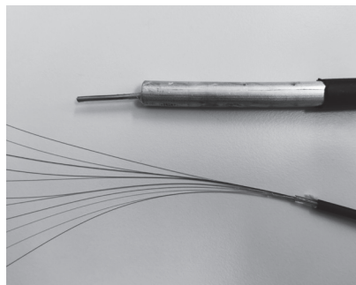
Ein Kupfer-Koaxialkabel (oben) im Vergleich zu einem Glasfaserkabel mit 12 Fasern (unten)
